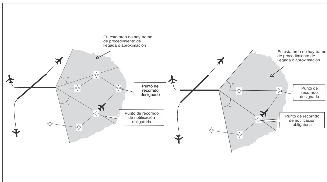
Figura 5-41. Área de protección de llegada
