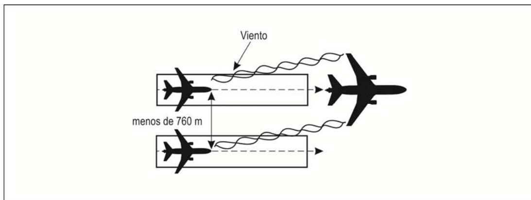
Figura 5-42. Separación por estela turbulenta para aeronaves que siguen [véanse 5.8.3.1 a) y b), y 5.8.3.2 a) y b)]
