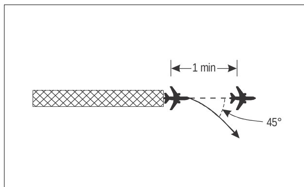
Figura 5-37. Separación de un minuto entre aeronaves que salen y siguen derrota divergentes por lo menos en 45° (véase 5.6.1)
