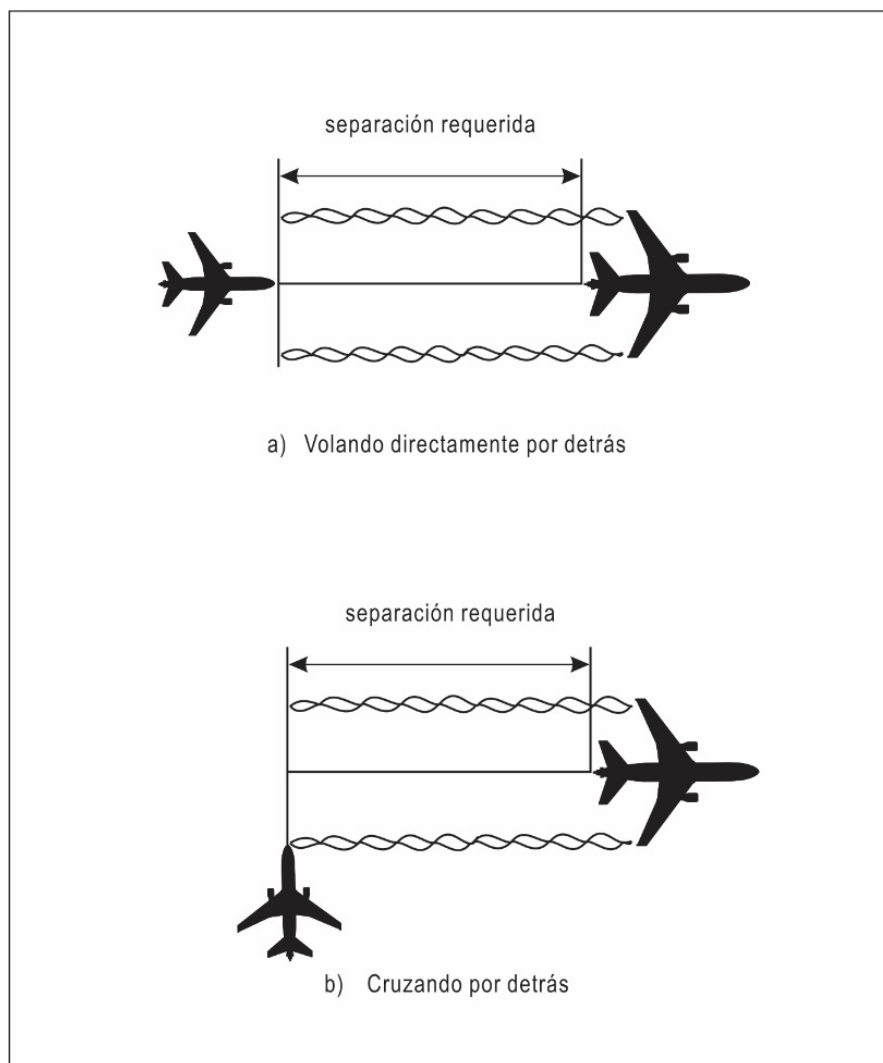
Figura 8-1. Vuelo directamente por detrás o cruce por detrás (véanse 8.7.3.4 y 8.7.3.5)
