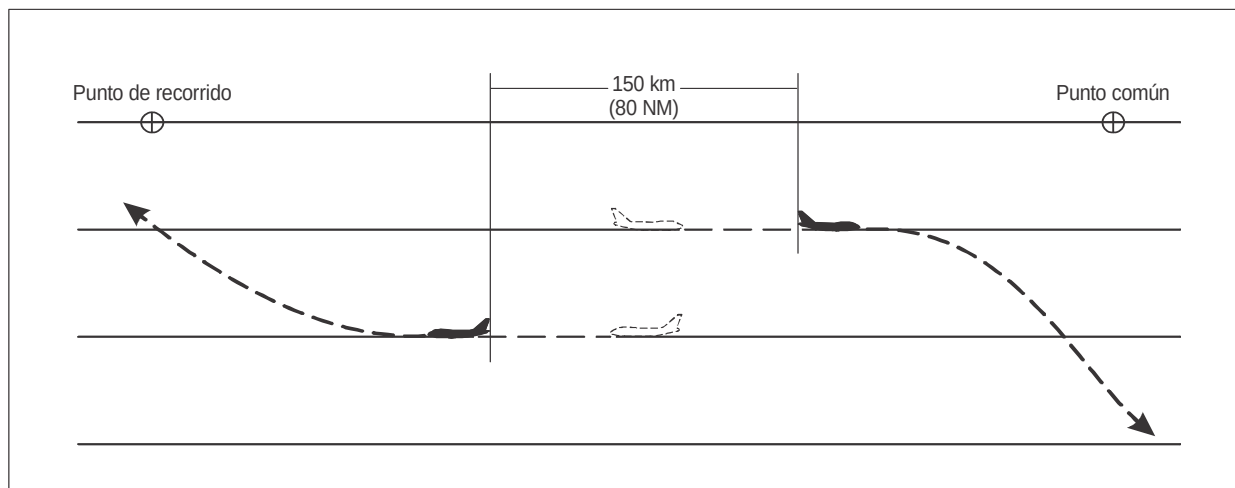
Figura 5-28. Separación de 150 km (80 NM) basada en RNAV entre aeronaves por derrotas opuestas (véase 5.4.2.5.7)
