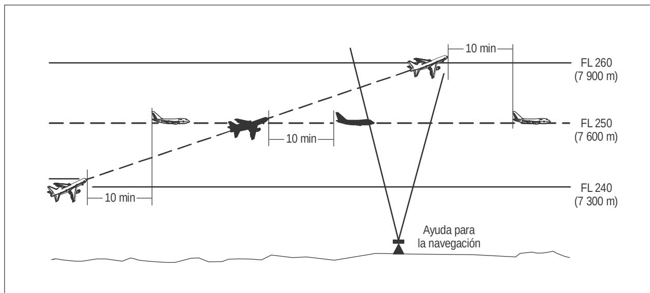
Figura 5-20A. Separación de 10 minutos entre aeronaves que ascienden y por derrotas que se cruzan [véase 5.4.2.2.2 b)]
