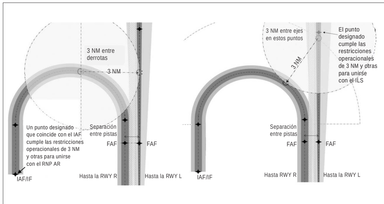
Figura 6-6. El concepto de ‘Establecida en la RNP AR APCH’ (Ejemplo de una aproximación RNP AR APCH/de precisión con una separación mínima de 3 NM)
