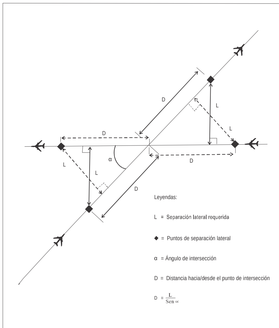
Figura 5-6. Puntos de separación lateral (véase 5.4.1.2.1.7)
