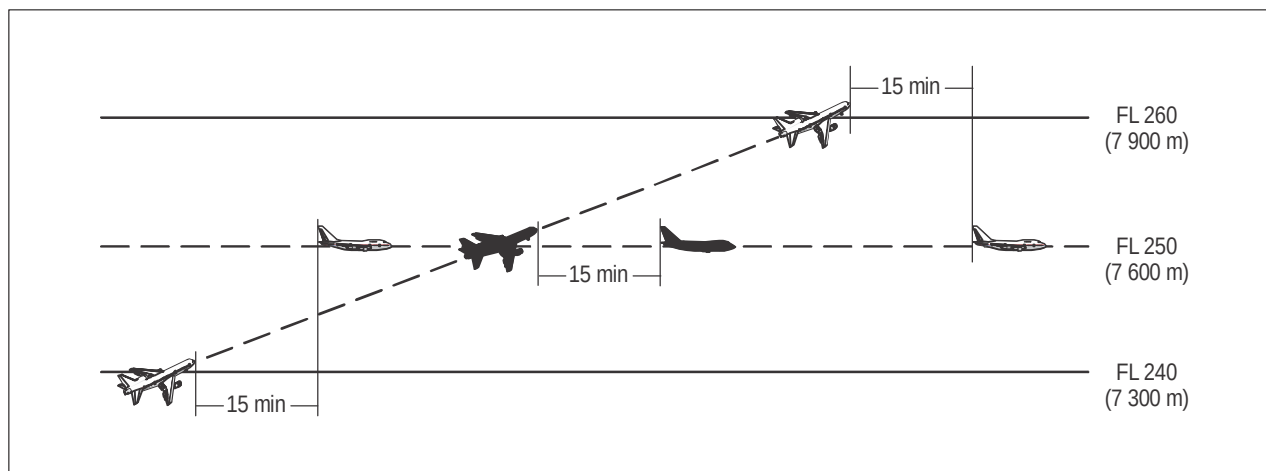
Figura 5-19A. Separación de 15 minutos entre aeronaves que ascienden y por derrotas que se cruzan [véase 5.4.2.2.2.2 a)]
