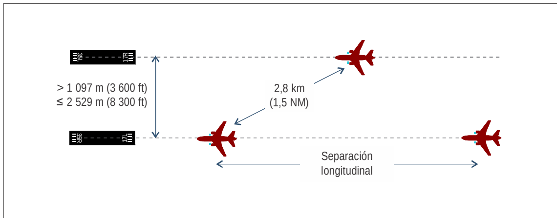
Figura 6-4. Separación diagonal para una distancia entre ejes mayor que 1 097 m (3 600 ft), pero menor o igual a 2 529 m (8 300 ft)
