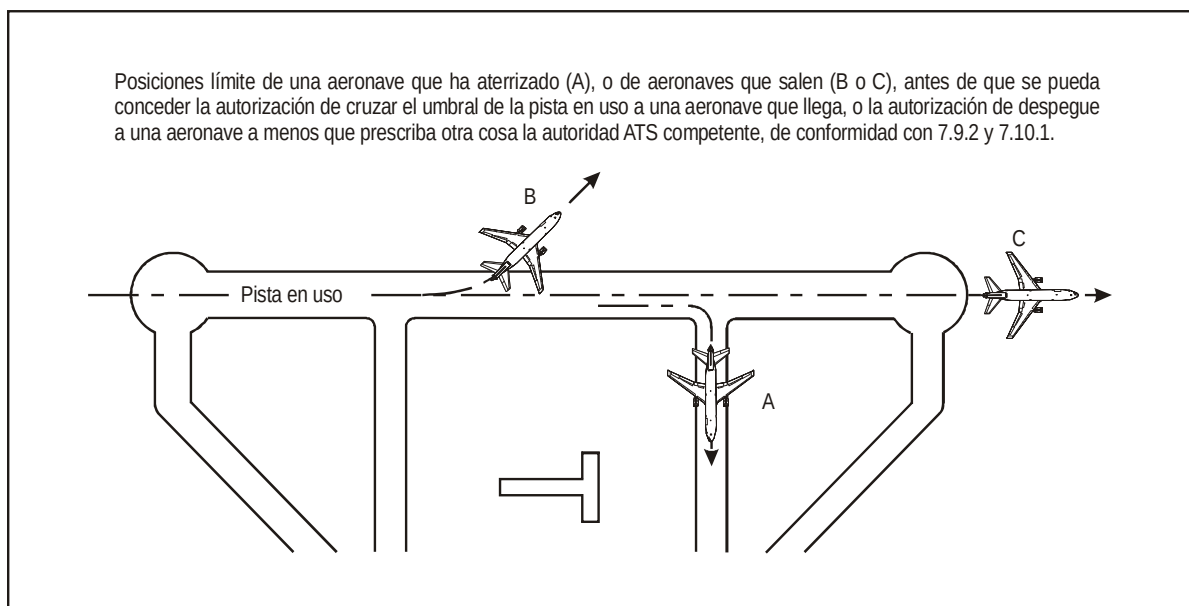
Figura 7-2. Separación entre aeronaves que llegan y salen (véanse 7.9.2 y 7.10.1)
