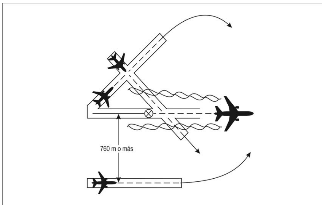
Figura 5-43. Separación por estela turbulenta para aeronaves que se cruzan [véanse 5.8.3.1 c) y d) y 5.8.3.2 c) y d)]
