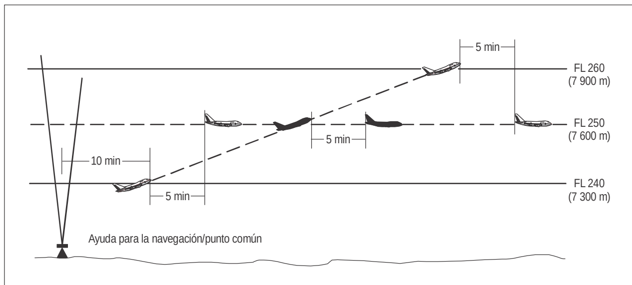
Figura 5-18A. Separación de cinco minutos entre aeronaves que ascienden y por la misma derrota [véase 5.4.2.2.1 c) 2)]
