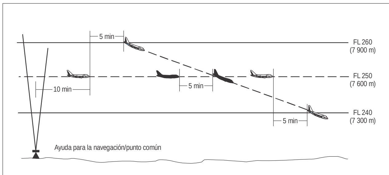
Figura 5-18B. Separación de cinco minutos entre aeronaves que descienden y por la misma derrota [véase 5.4.2.2.1 c) 2)]
