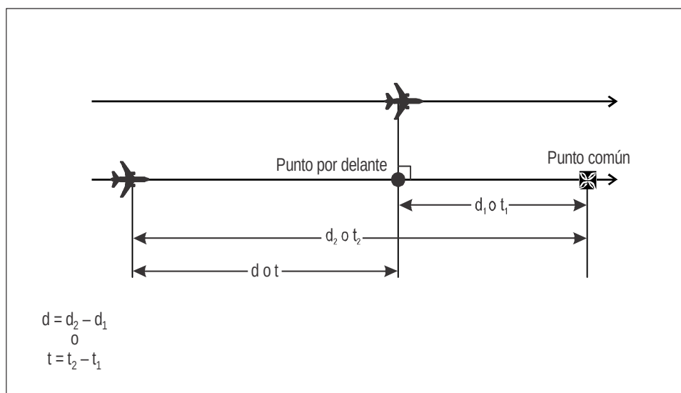
Figura 5-35. Cálculo de la distancia/tiempo longitudinal entre aeronaves — derrota paralelas [véase 5.4.2.9.5 c)]
