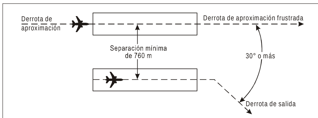
Figura 6-7. Operaciones paralelas segregadas [véase 6.7.3.6.1 b)]
